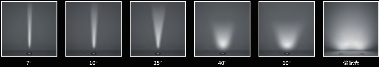
多种不同的配光角度选择 Different options of beam angle light distribution
